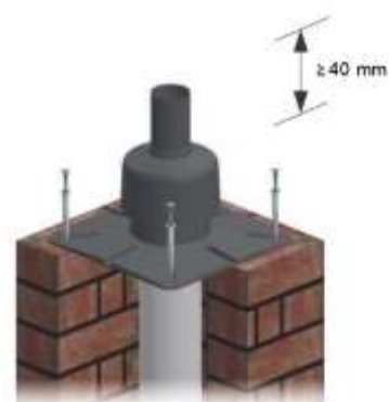
Abdeckplatte fest dübeln. Bei Bedarf den Kopf mit einer Betonabdeckung verstärken!
