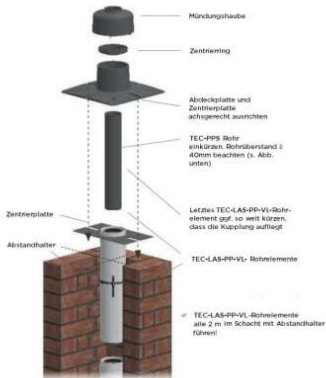
Abb. zeigt Montagebeispiel für Luft-Abgassystem TEC-LAS-PP-VL
