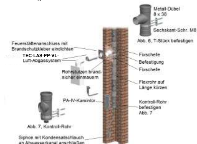
Abb. 8, unterer Leitungsabschnitt mit 1. Feuerungsanschluss
