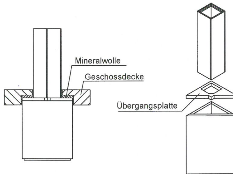
Übergang in Geschossdecke
