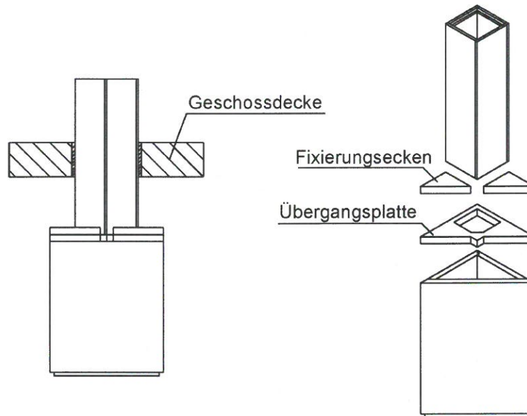
Übergang unter Geschossdecke mit Fixierungsecken
